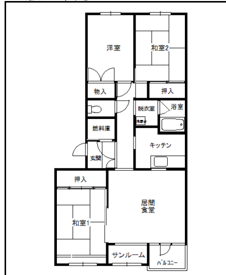
(反転タイプあり) 3LDK (2,3,6,7,10,11号室)
