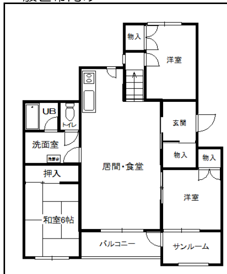
(反転タイプあり) 3LDK (3～9, 13～18号室)
