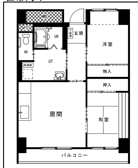
反転タイプあり 2LDK
